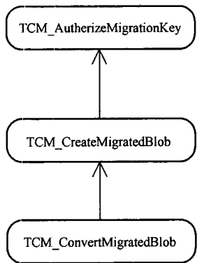
图 12 密钥迁移命令依赖关系
