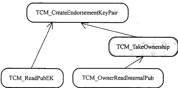
图 7 TCM 背书密钥管理命令依赖关系
