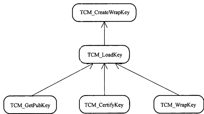
图 10 密钥管理命令依赖关系
