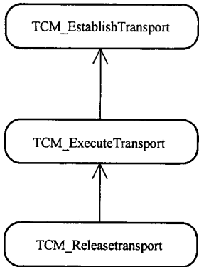
图 14 传输会话命令依赖关系
