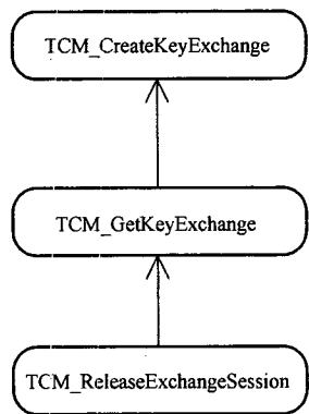
图 11 密钥协商命令依赖关系
