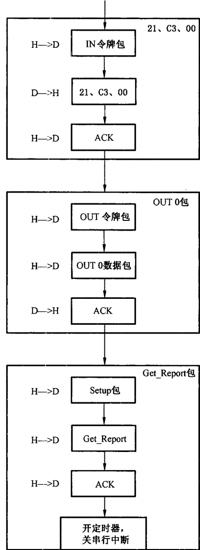
图 10 HID 设备数据延时处理流程
