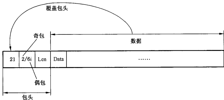
图 8 HID 设备数据包装示意图
