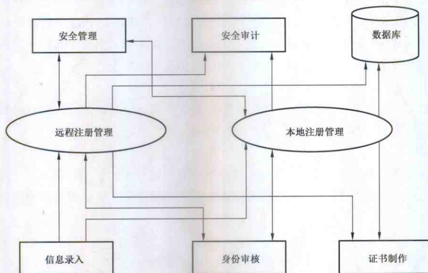
图 2 用户注册管理系统逻辑结构
