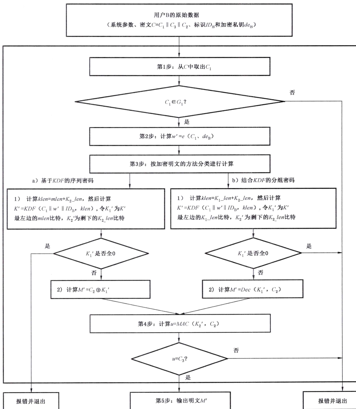
图4 解密算法流程
